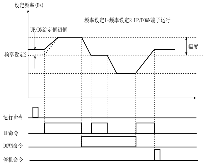
图 5-3-3 UP/DOWN 端子组合运行
