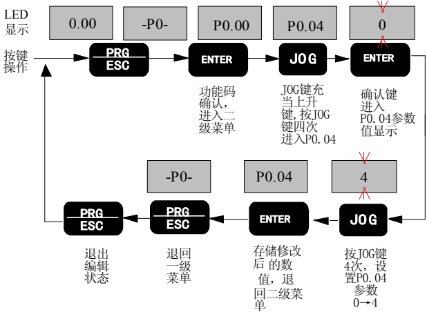
图 3-8 UP/DN 使能操作示例
