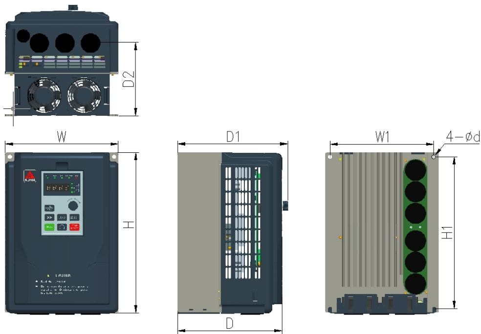
附录1 外型尺寸与安装尺寸（单位：mm）
