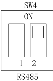
图 2-13 RS485匹配电阻拨码开关示意图
