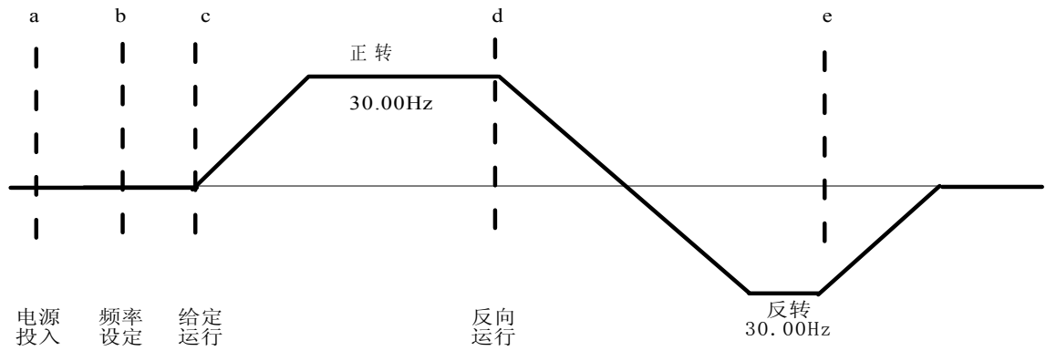
图 3-12 键盘运行时序图
