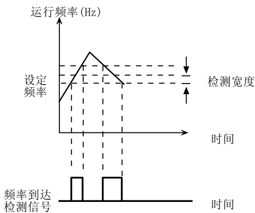
图 5-3-8 频率到达检测
