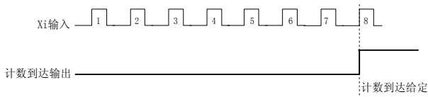
图 5-3-12 计数到达
