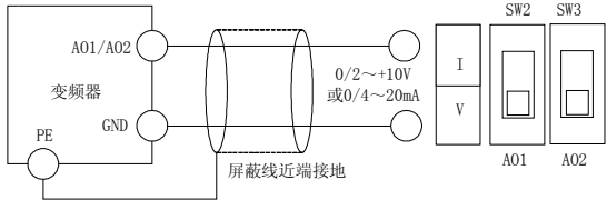
图 2-10 模拟输出端子配线图
