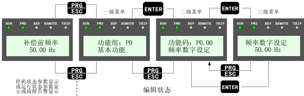
图 A6-3 LCD 键盘的编程显示状态
