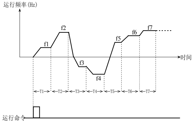
图 5-5-2 PLC 单循环后保持方式
