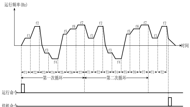
图 5-5-3 PLC 连续循环方式
