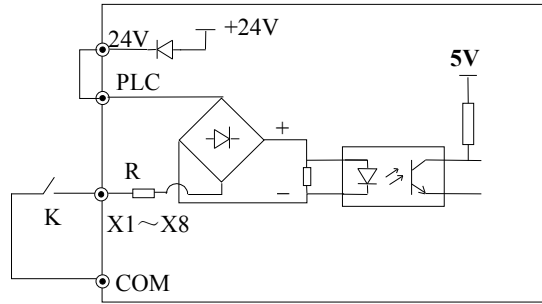
图 2-14 使用内部24V电源的连线方式
