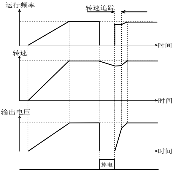
图 5-1-2 转速追踪
