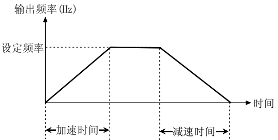
图 5-1-4 直线加减速
