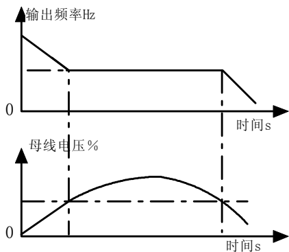
图 5-13-5 减速过程
