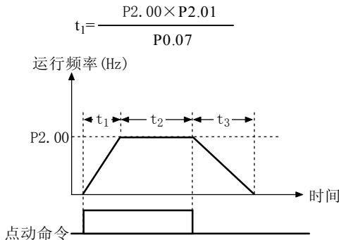
图 5-2-1 点动运行参数说明
