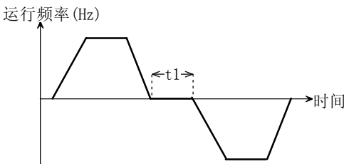
图 5-2-2 正反转死区时间
