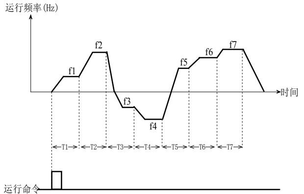
图 5-5-1 PLC 单循环后停机方式
