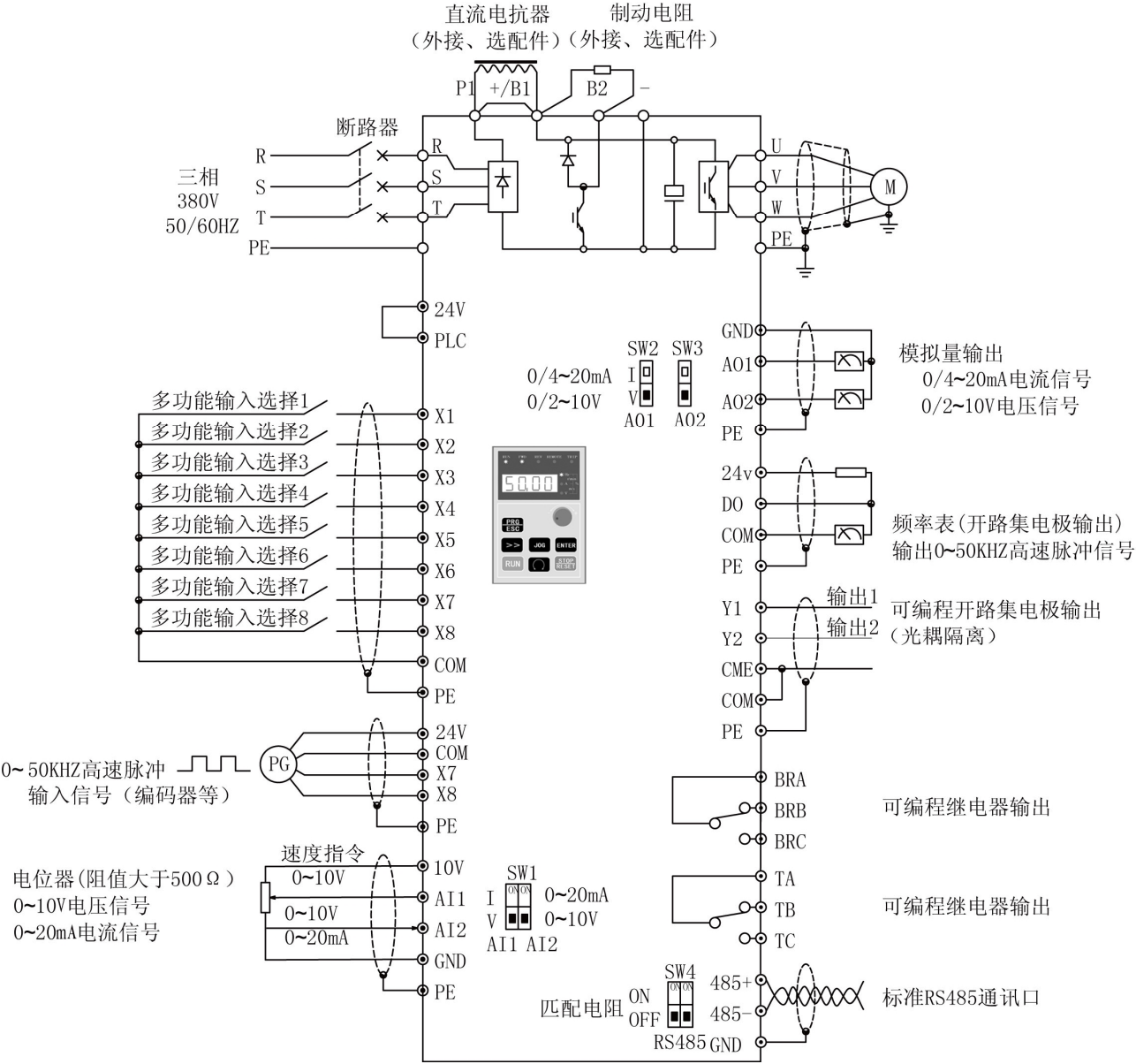
图 2-25 35R5GB/37R5PB~3015GB/3018PB 接线图
