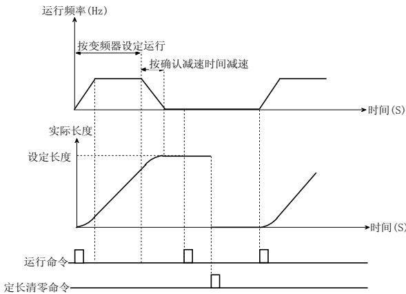
图 5-8-1 定长运行
