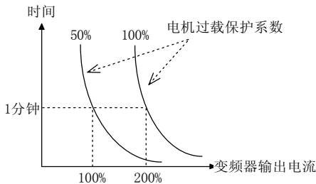
图 5-13-1 电机过载保护系数设定
