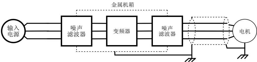
图 2-7 射频干扰抑制措施图
