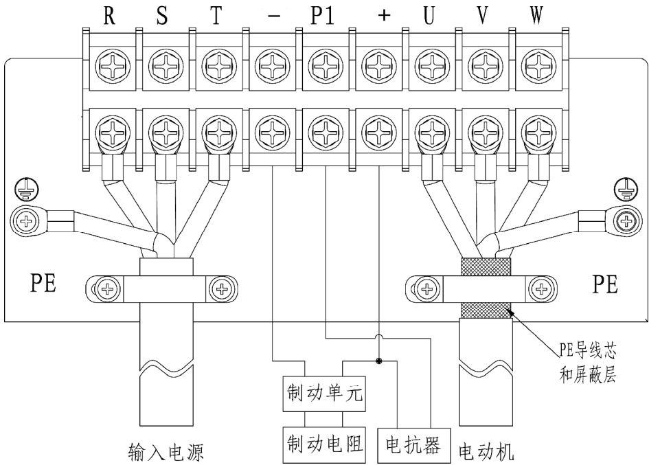
图 2-3 3018G/3022P~3132G/3160P 机型主回路端子接线
