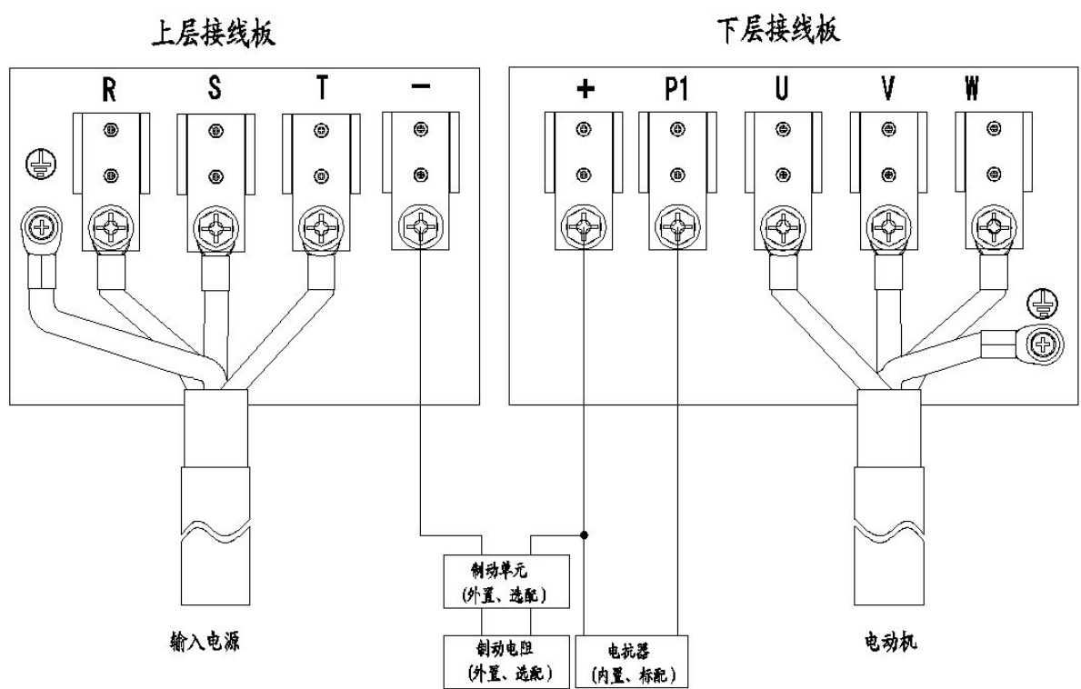
图 2-5 3400G~3500G 机型主回路接线端子
