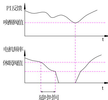
图 5-7-3 休眠和唤醒
