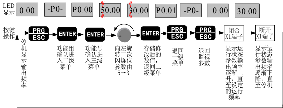
图 3-16 端子运行与停机的操作示例
