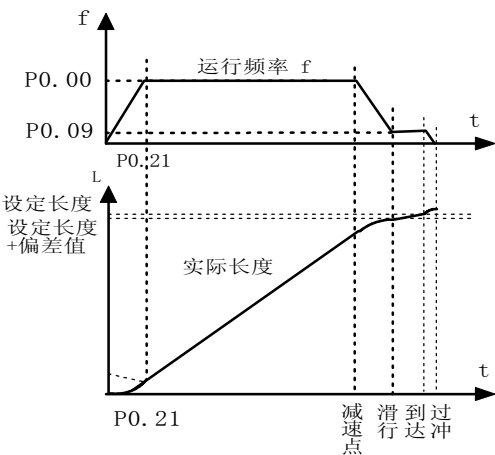
图 5-8-2 定长运行2
