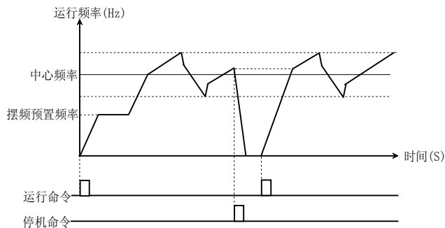
图 5-6-2 摆频起动：按停机前状态
