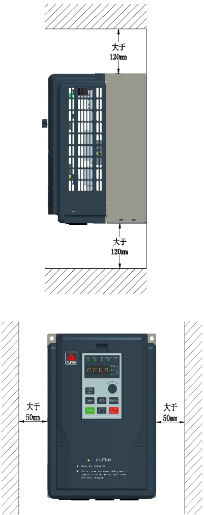
图 2-1 安装方向和空间
