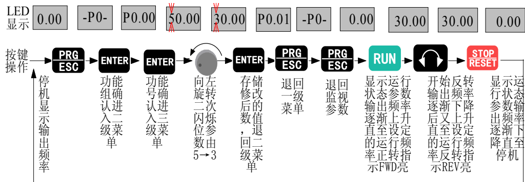
图 3-13 运行与停机的操作示例
