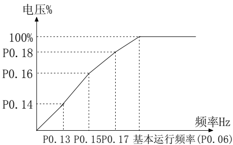
图 5-0-3 用户设定V/F曲线一般形式
