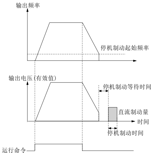
图 5-1-6 停机制动
