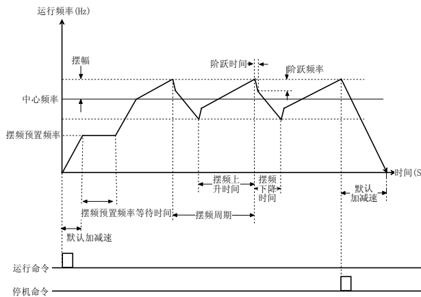
图 5-6-1 摆频示意图
