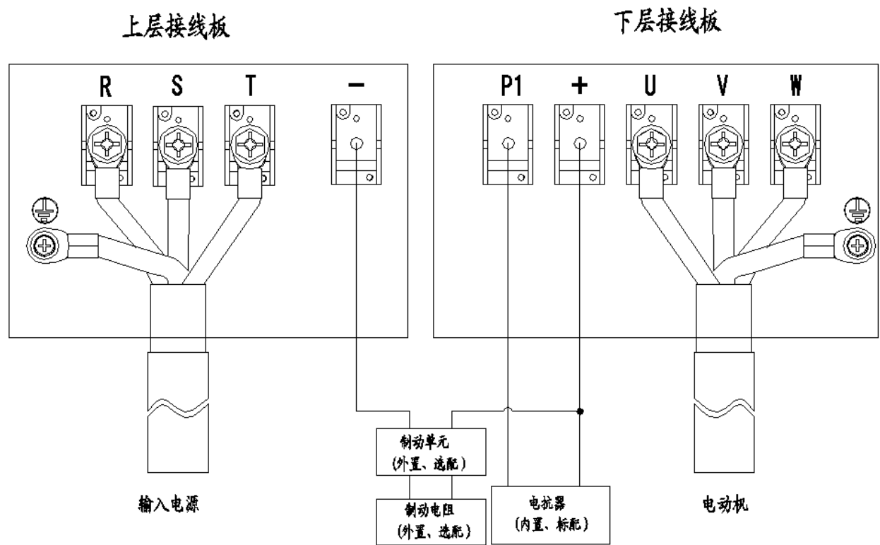
图 2-4 3160G/3200P~3355G/3400P 机型主回路接线端子
