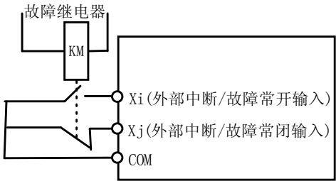
图 5-3-6 常开/常闭
