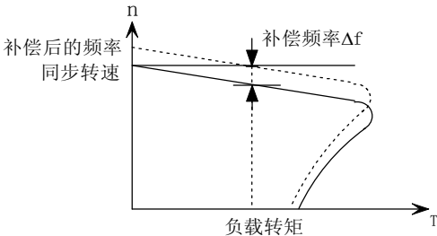
图 5-9-1 自动转差补偿
