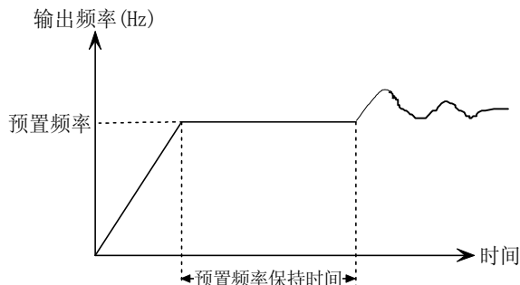
图 5-7-2 PID 预置频率运行示意图
