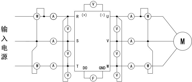
图 8-1 主回路电气测量的推荐接法
