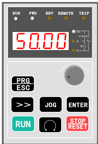
图4 运行状态，RUN灯亮， 运行到设定频率 稳速时FWD恒亮
