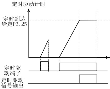
图 5-3-7 定时驱动输入
