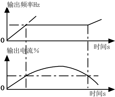
图 5-13-3 加速过程
