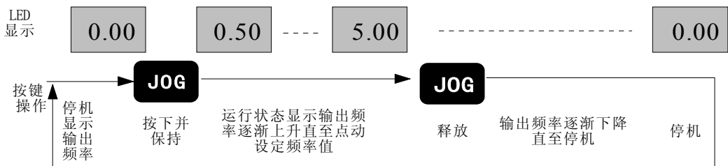
图 3-14 点动运行的操作示例
