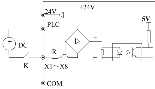
图 2-15 使用外部电源的连线方式
