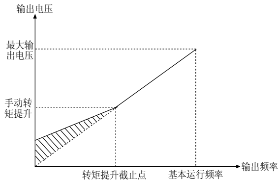
图 5-0-4 手动转矩提升（提升量为阴影部分）
