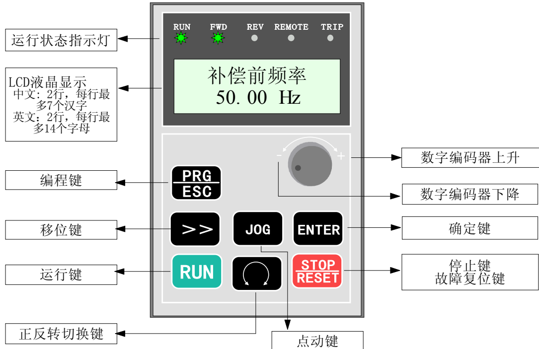
图 A6-1 LCD 键盘布局与各部分名称
