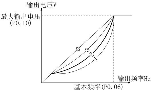
图 5-0-2 降转矩曲线
