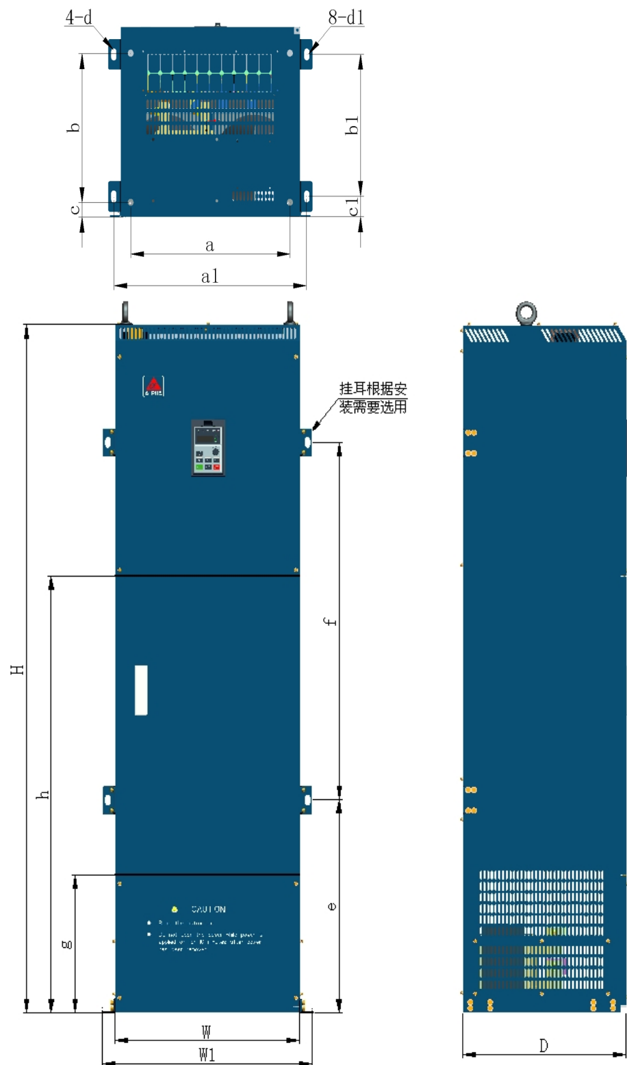
附录 1 外型尺寸与安装尺寸
