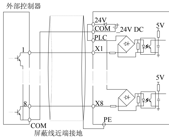
图 2-16 使用变频器内部+24V电源的源极连接方式
