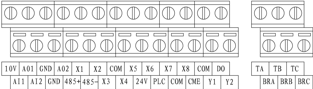
图 2-8 控制回路端子排布
