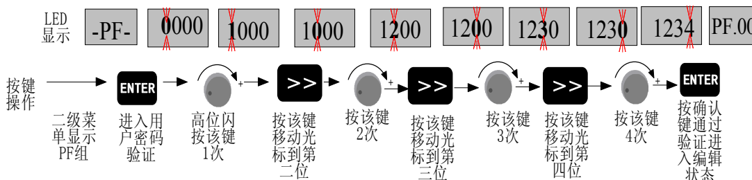
图 5-15-2 用户密码解锁流程
