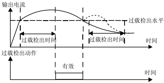
图 5-13-2 过载预警检出功能示意图
