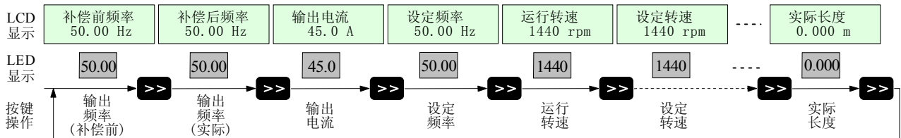
图 A6-5 LCD 键盘：监视参数显示操作示例
