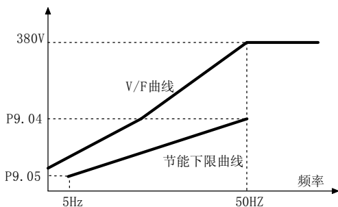
图 5-9-2 节能电压下限限制
