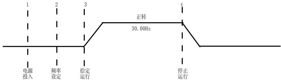
图 3-15 端子运行时序图
