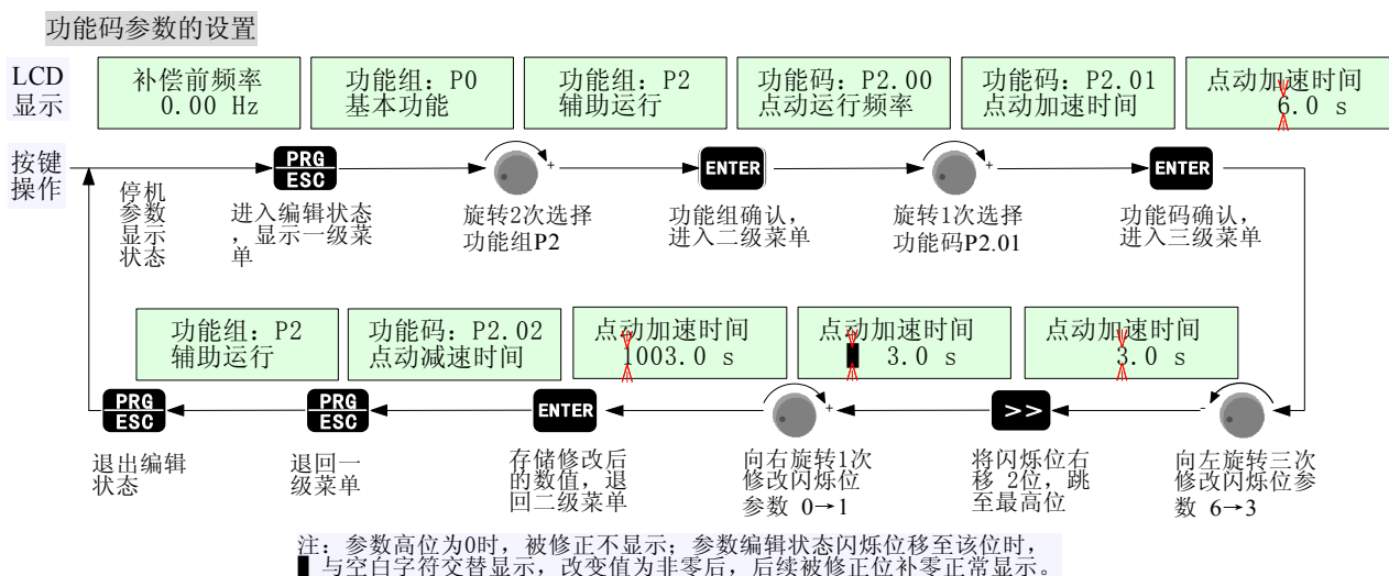
图 A6-7 LCD 键盘：参数编辑操作示例
