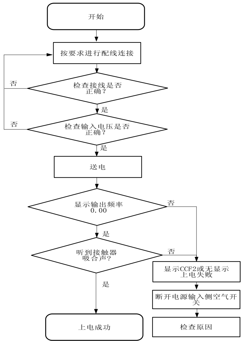
图 3-11 变频器初次上电操作流程
