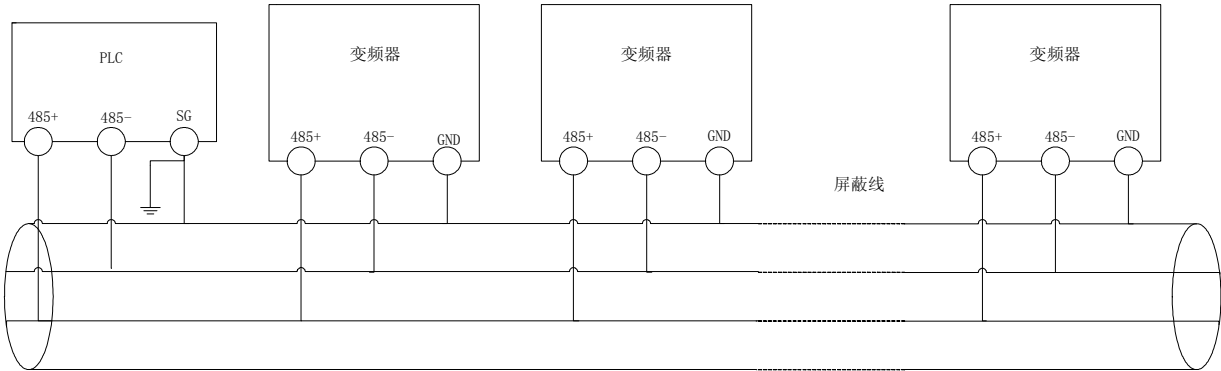
图 2-12 PLC与变频器多机通信时推荐的接线图（变频器、电机全部良好接地）
