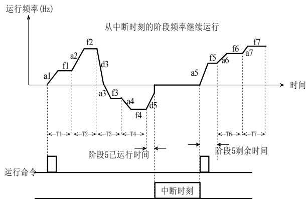
图 5-5-4 PLC 起动方式 1
