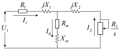
图 5-10-1 异步电机稳态等效电路图
