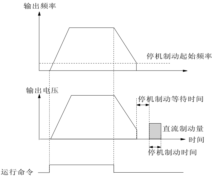
图 5-3-5 停机直流制动
