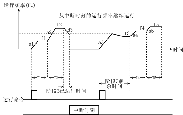
图 5-5-5 PLC 起动方式 2
