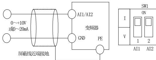
图 2-9 模拟输入端子配线图
