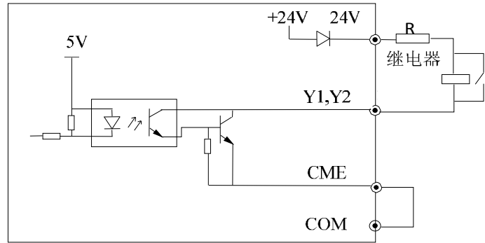
图 2-20 多功能输出端子接线方式1
