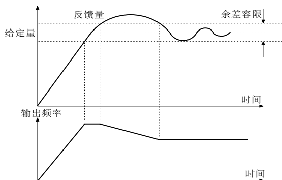
图 5-7-1 余差容限示意图
