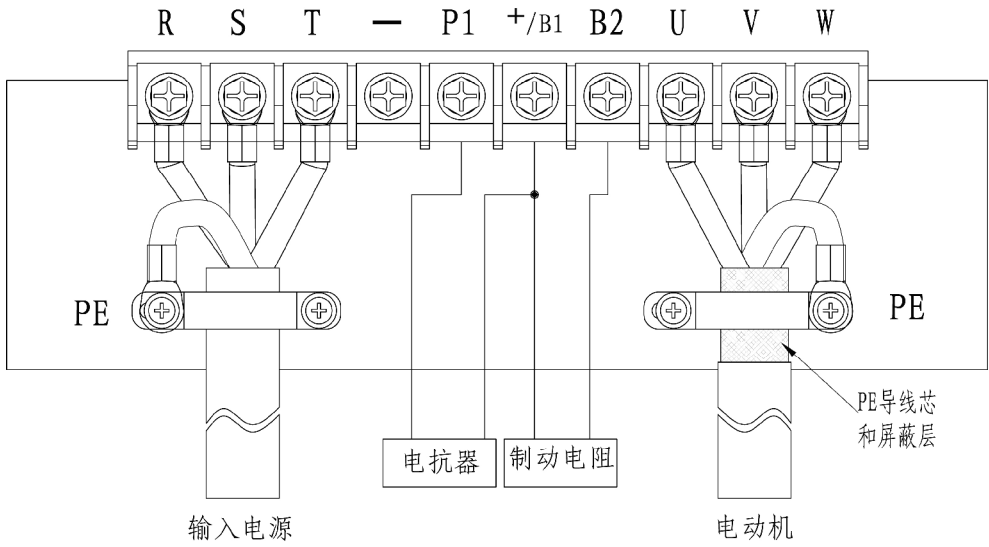
图 2-2 35R5GB/37R5PB~3015GB/3018PB 机型主回路端子接线
