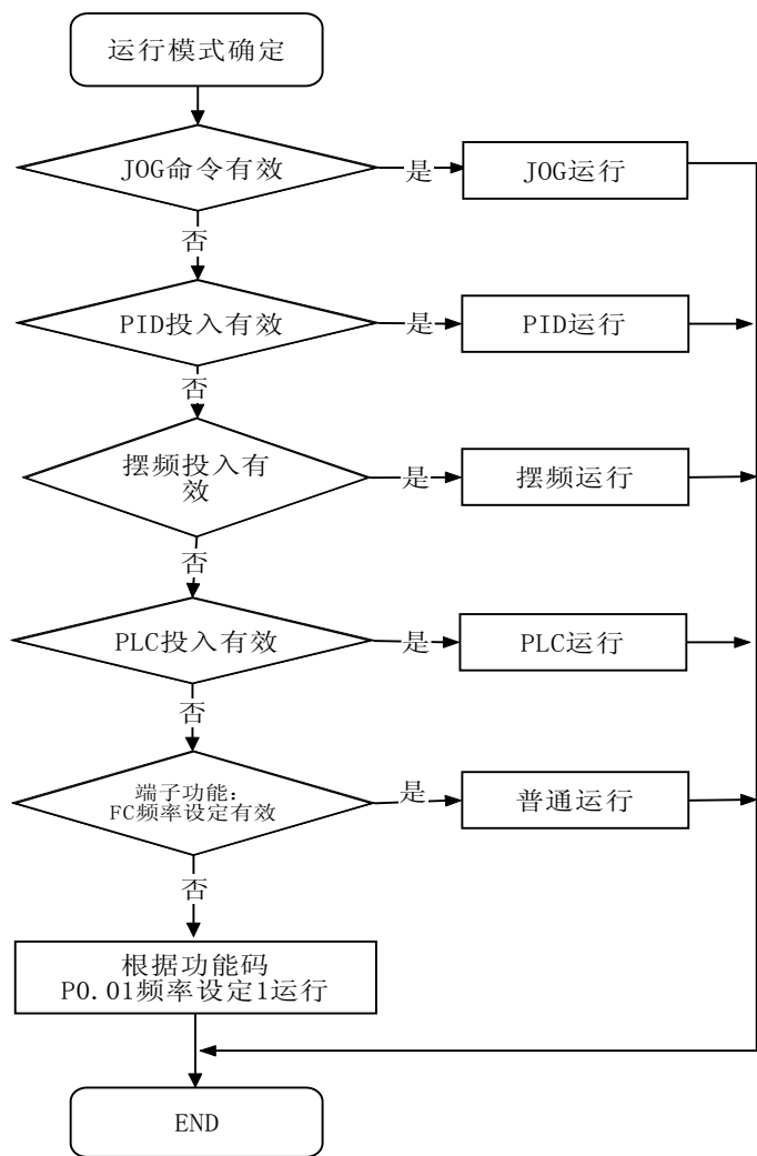
图 3-10 变频器运行状态切换流程
