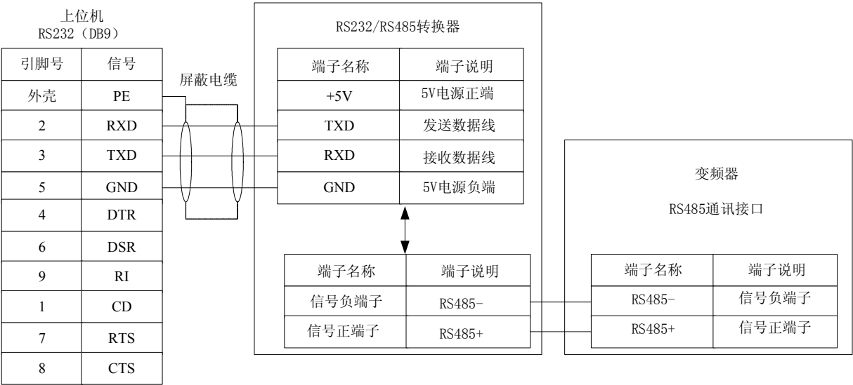
图 2-11 上位机与变频器接口接线图
