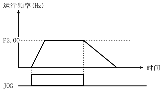
图 5-3-2 JOG运行
