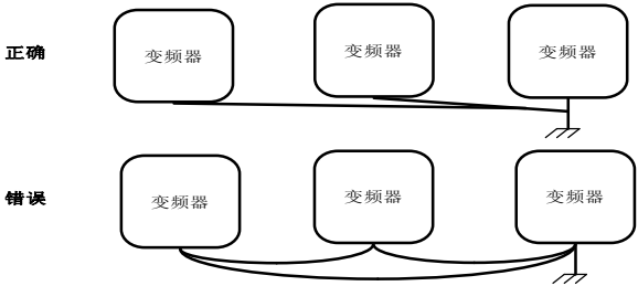
图 2-6 接地线连接方法
