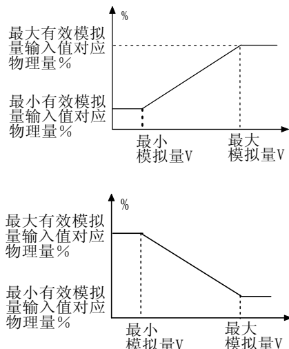
图 5-4-1 模拟输入线性曲线
