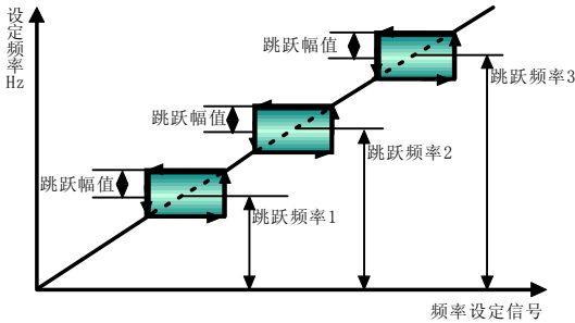
图 5-2-5 跳跃频率
