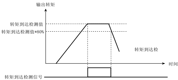
图 5-3-11 转矩到达检测
