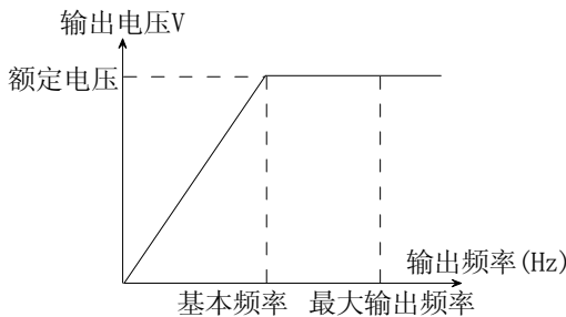
图 5-0-1 输出频率与输出电压关系图
