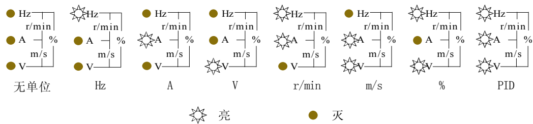
图 3-2 单位指示灯状态与单位对应关系图
