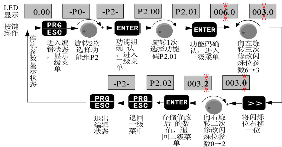
图 3-7 参数编辑操作示例
