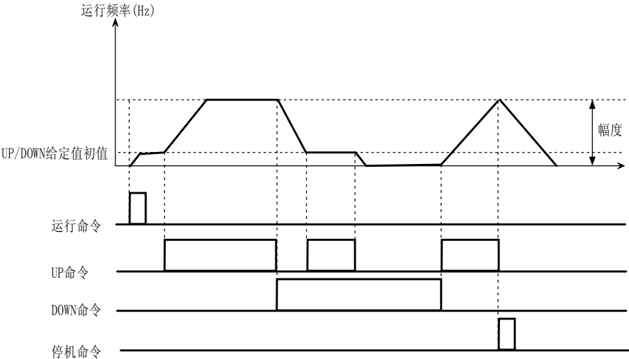
图 5-3-4 UP/DOWN 端子非组合运行
