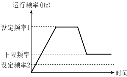
图 5-2-3 运行在下限频率
