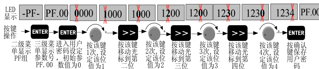
图 5-15-1 用户密码设定流程
