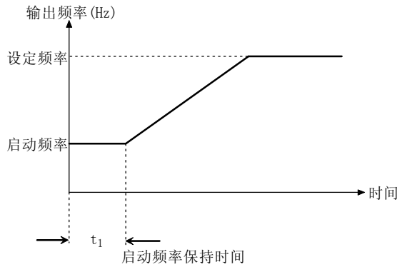
图 5-1-3 启动频率与启动时间示意图
