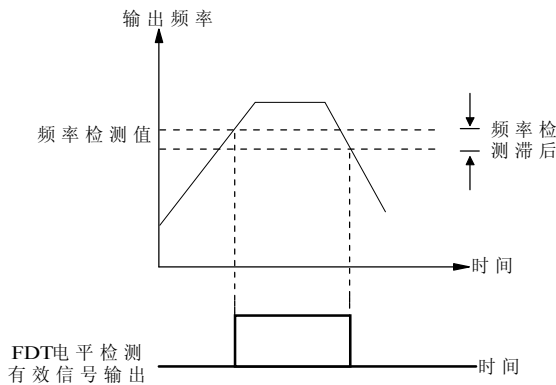
图 5-3-9 频率检测FDT
