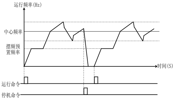
图 5-6-3 摆频启动：重新开始
