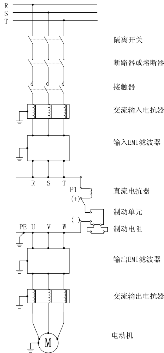
图 7-1 外围设备连接图
