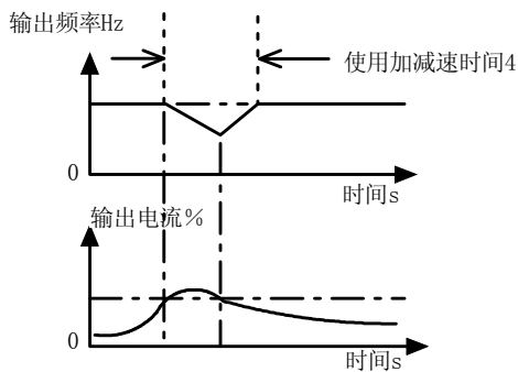
图 5-13-4 稳定运行过程
