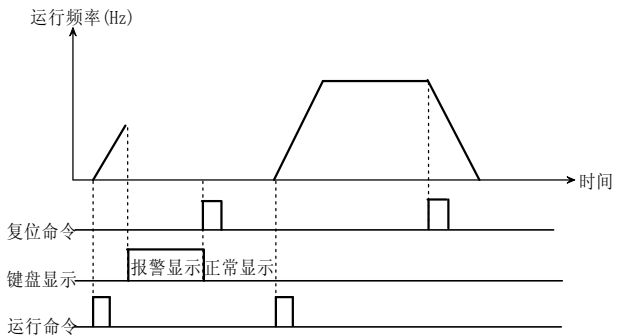
图 5-3-1 端子复位
