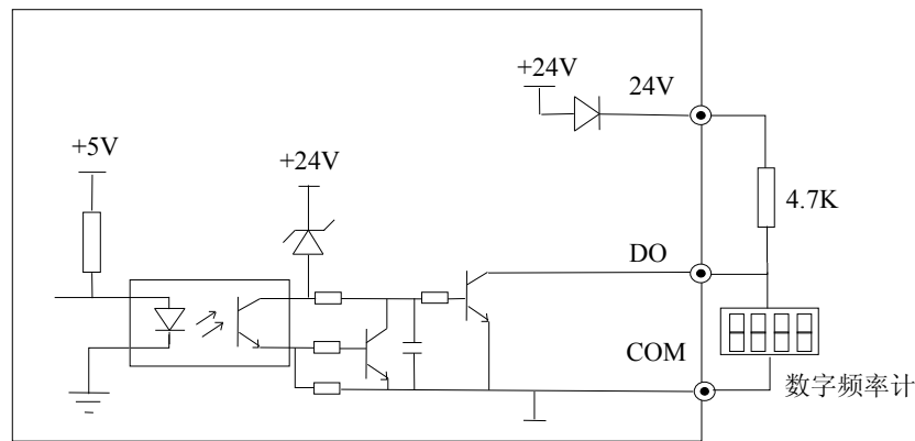
图 2-22 输出端子DO连接方式1
