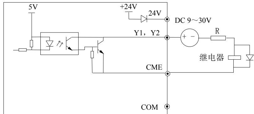
图 2-21 多功能输出端子接线方式2
